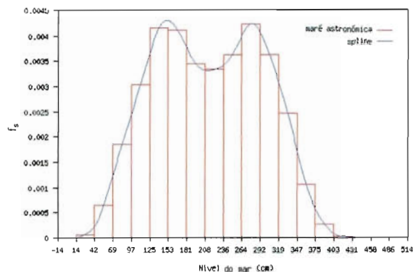
Figura 4.12 – Ajuste de spline cúbica à série da maré astronômica, com base em 14 anos de dados, para o porto de Viana do Castelo
