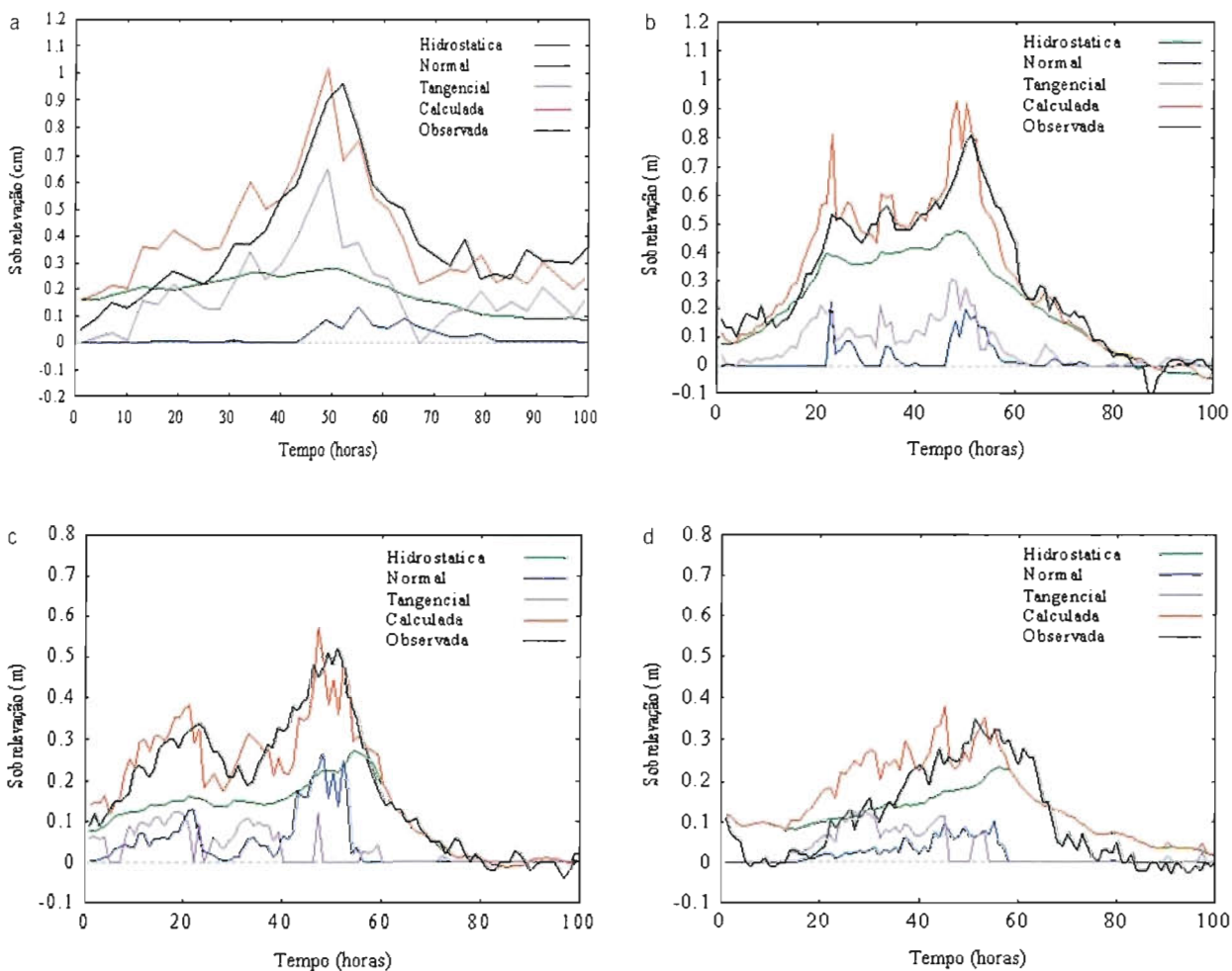
Figura 4.15 Representação gráfica de episódios em que se observaram máximos anuais da sobrelevação nos marégrafos dos portos em análise: A – Viana do Castelo (1979); B – Leixões (1982); C – Cascais (1987); D – Lagos (1988)
