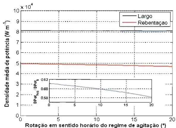
Figura 4.43 – Variação da densidade média de potência em função da rotação do regime de agitação ao largo. O encaixe pormenoriza os resultados na rebentação ( DPot_{Reb} ) normalizados pelos valores ao largo ( DPot_{L} )
