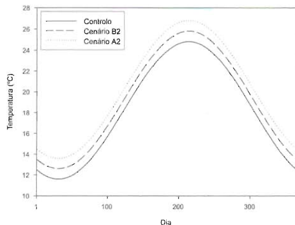
Figura 10.55 Variação da temperatura ao longo do ano num tanque de aquicultura do estuário do Sado, de acordo com a situação de controlo, baseada nos dados de Ribeiro et al. (2000) e os cenários B2 e A2
