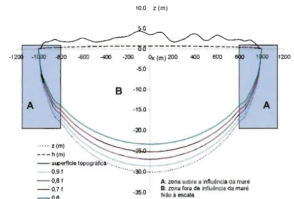
Figura 3.41 – Estimativa da espessura da lente de água doce no aquífero superior da península de Tróia: Situação com a recarga actual, e com recargas efectivas de 90 %, 80 %, 70 % e 60 % da actual
