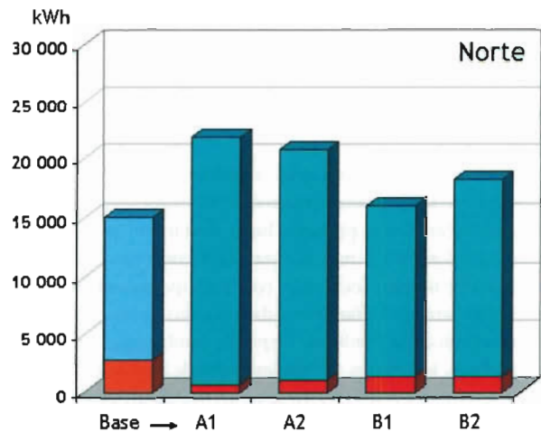
Figura 7.11 – Impacto das alterações climáticas no consumo de energia para climatização em escritórios no Norte do país (aquecimento representado em laranja e vermelho e arrefecimento em tons de azul).
