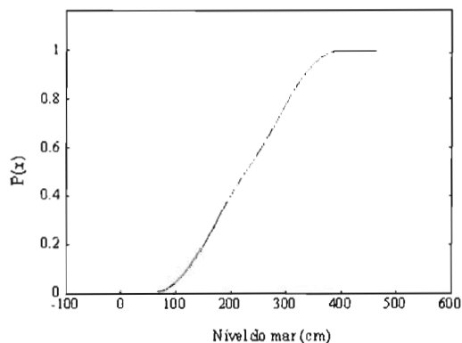
Figura 4.13 – Representação gráfica da convolução entre as séries da sobrelevação do nível do mar e da maré astronômica para o porto de Lagos
