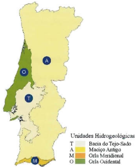
Figura 3. 2 – Unidades hidrogeológicas
