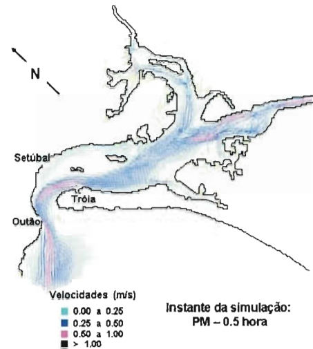
Figura 10.46 – Campos de velocidade instantânea em maré viva simulados
