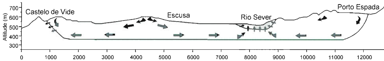
Figura 3.36 - Modelo conceptual do fluxo subterrâneo no aquífero de Escusa
